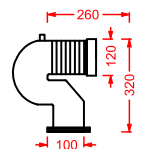
ART ACA034 CURVA TECNICA TRASLATA
