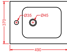
BKB001 BLOCK bidet sospeso wall-hung bidet
