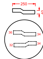
ART ACA035 CANNOTTO TRASLATO PER MODIFICA
