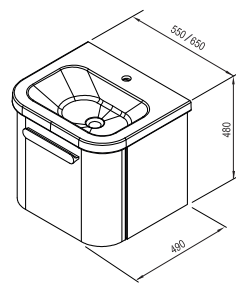
SD 550 / 650 Chrome
