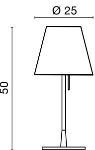
2111 2,9 kg 70W E27 ECO 21W E27 Fluo EL 10W E27 Led (cod. 0105) F □ .57
