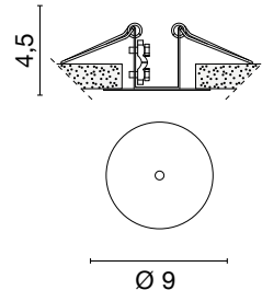
Piastra con molle per controsoffitti. Ceiling plate with springs.
